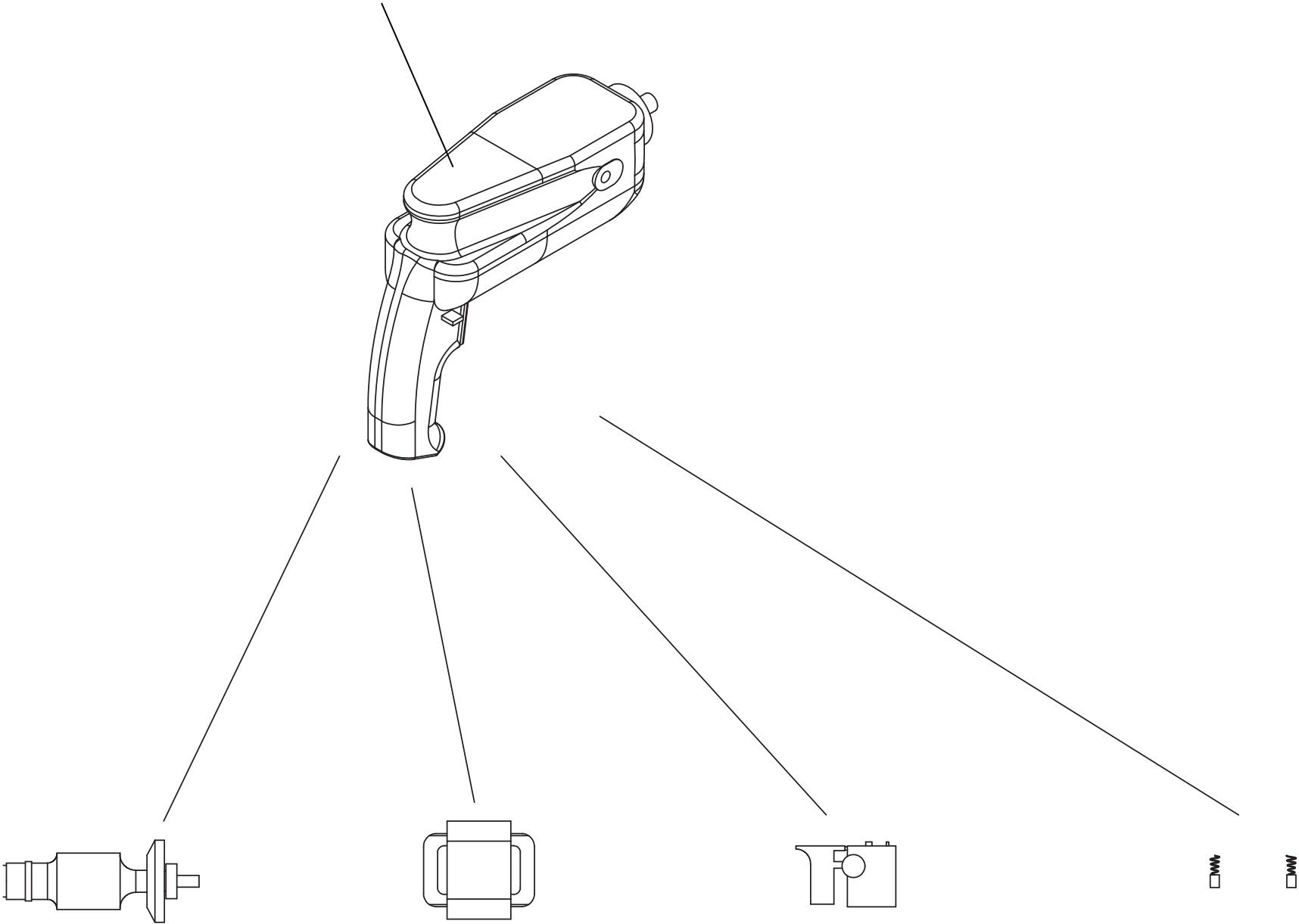
15、 D10VG HIKOKI Drilling Unit
